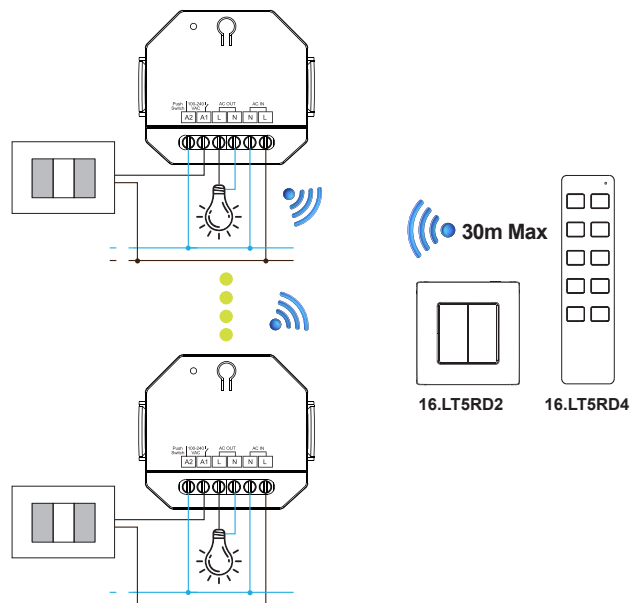
Schema collegamento
