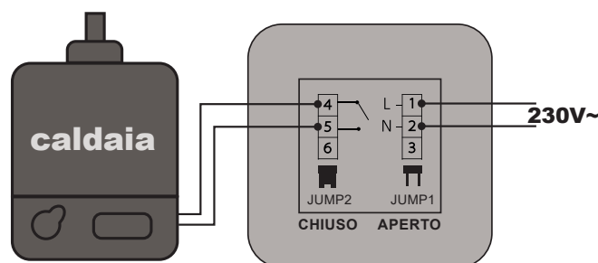
Modalità GC Esempio schema contatto pulito con caldaia
