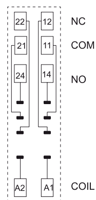
Schema collegamenti
