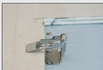
Particolare inserimento pannello
