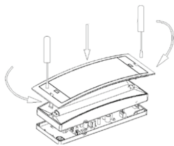
Esploso apparecchio d'emergenza
